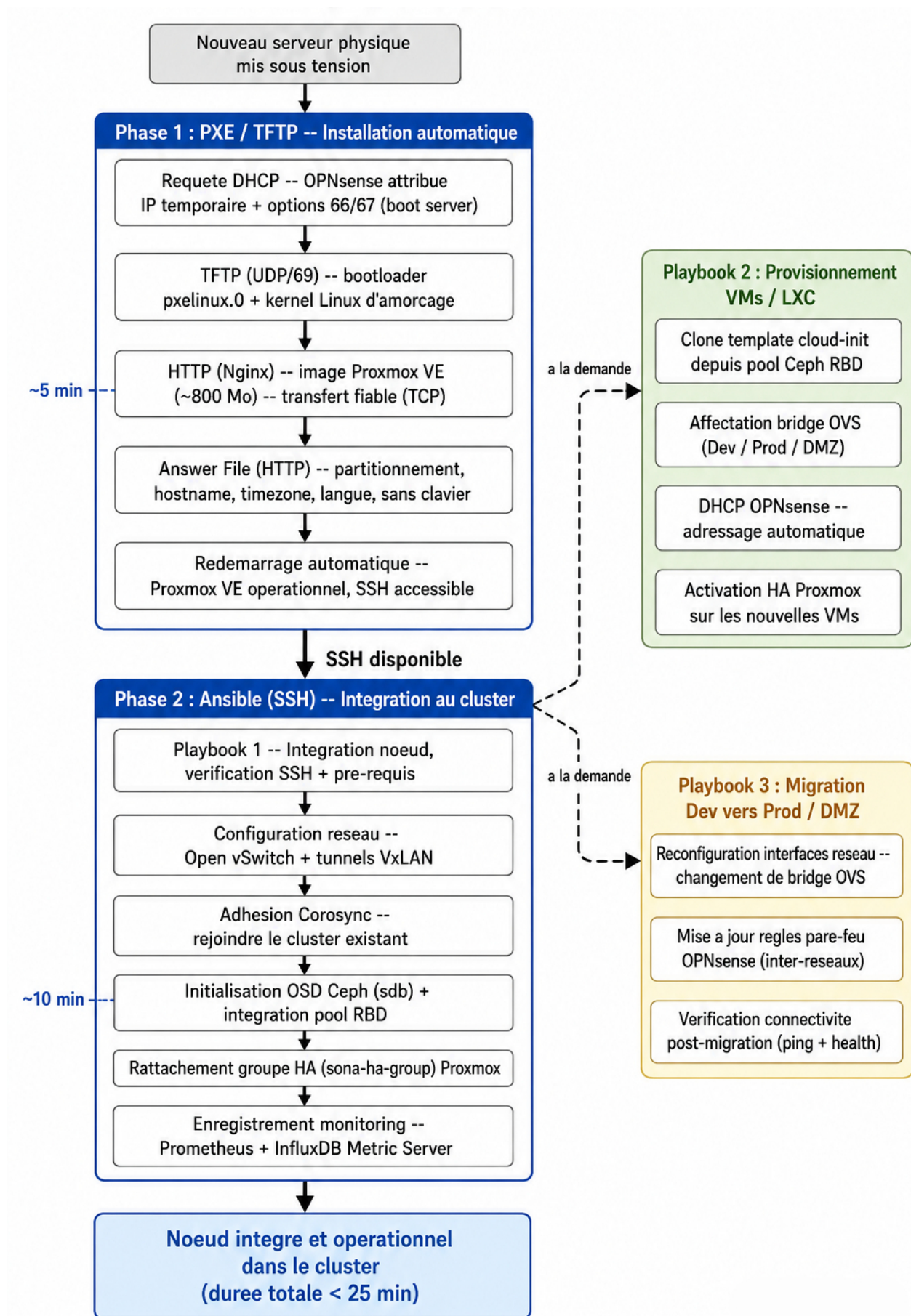
FIGURE III.6 – Pipeline d'Automatisation : PXE/TFTP et Ansible
